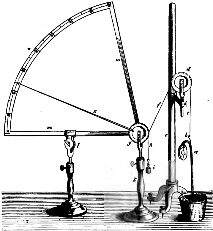
Fig. 449. — Indicateur sur arc. Appareil pour mesurer les allongements des entre-nœuds dans de courts intervalles de temps.
